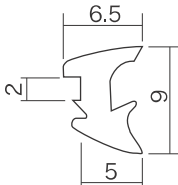
ガラスビート
