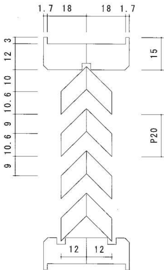
ドア厚36での基本寸法
