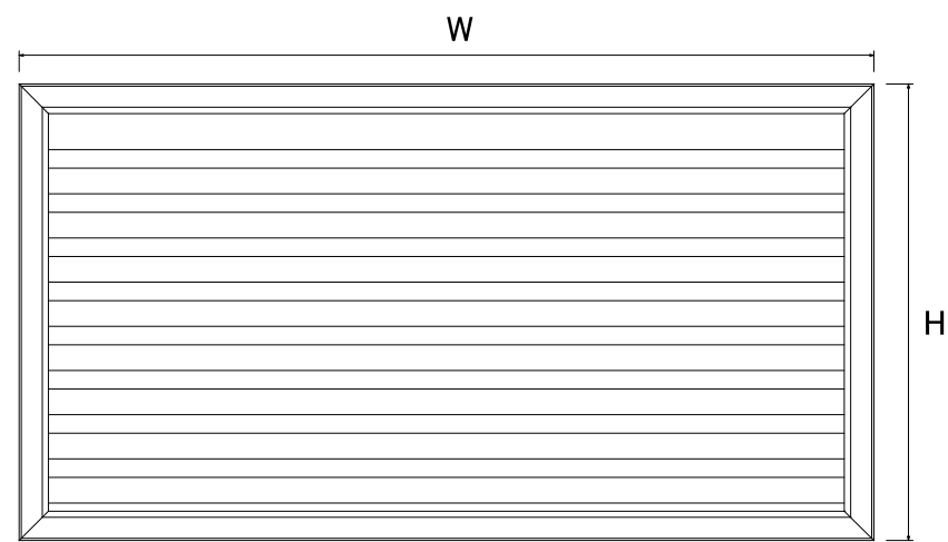
ドア厚36での基本寸法
